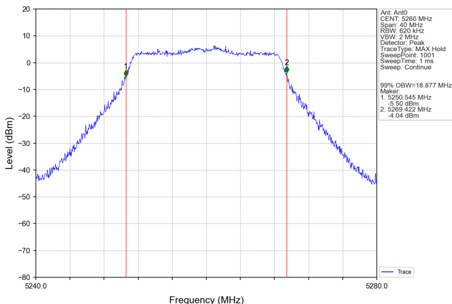
802.11ac(VHT20)_LCH_5260MHz_Ant0_NTNV
