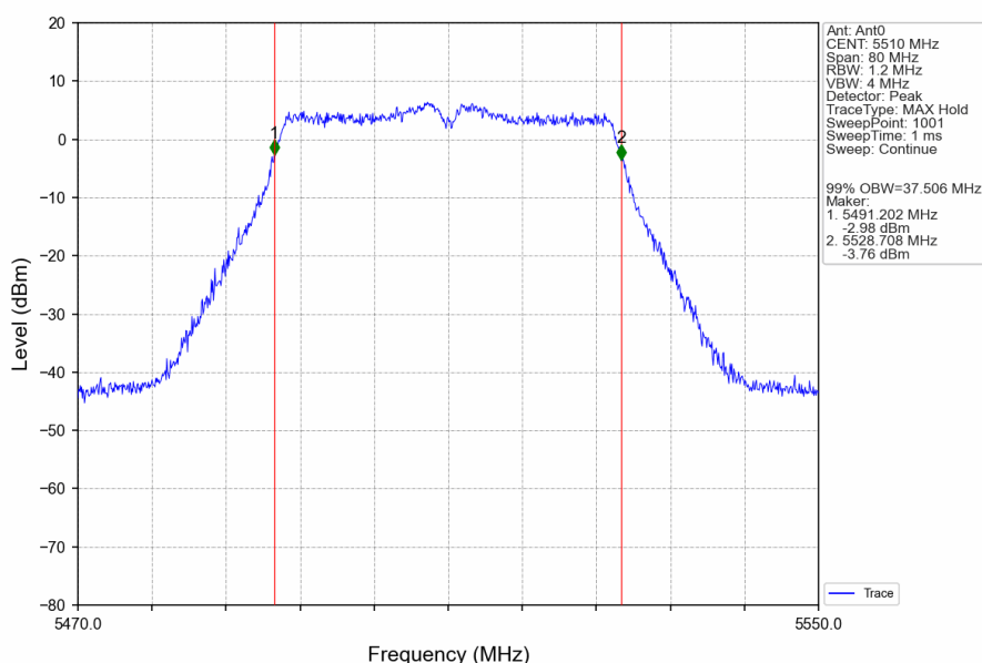
802.11ac(VHT40)_LCH_5510MHz_Ant0_NTNV
