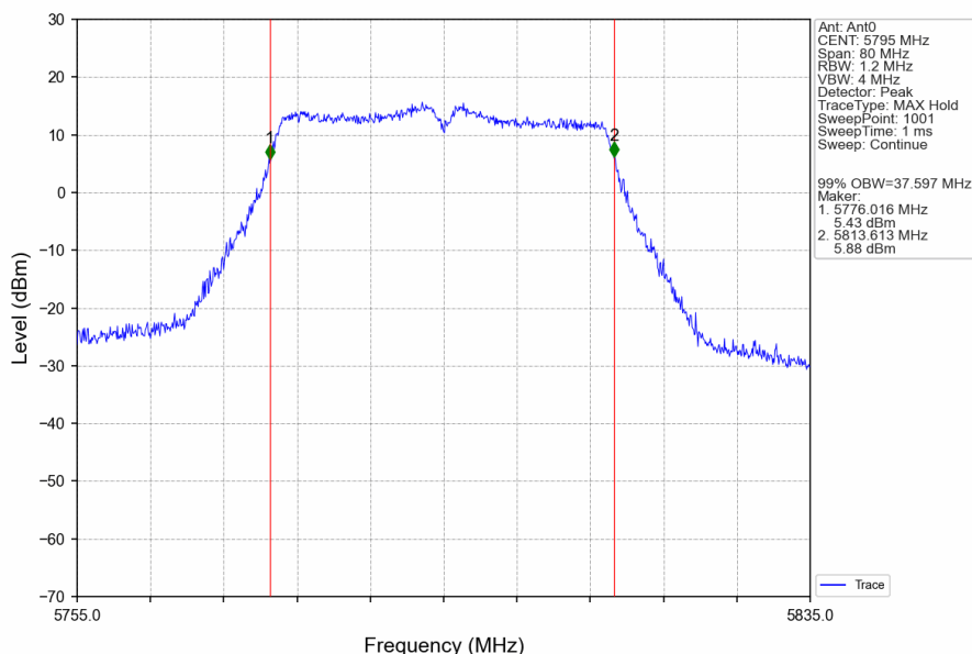
802.11ac(VHT40)_HCH_5795MHz_Ant0_NTNV
