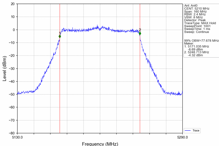
802.11ac(VHT80)_MCH_5210MHz_Ant0_NTNV
