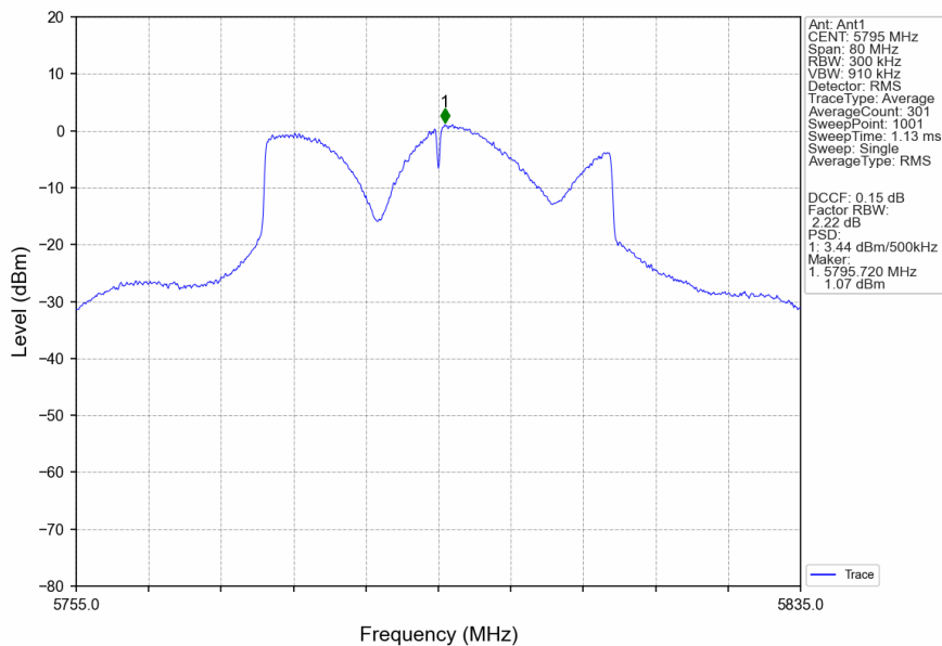
802.11be(EHT40)_HCH_5795MHz_SU_ / _Ant1_NTNV
