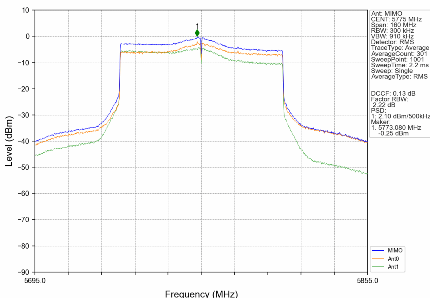
802.11ax(HEW80)_MCH_5775MHz_SU_ / _MIMO_NTNV
