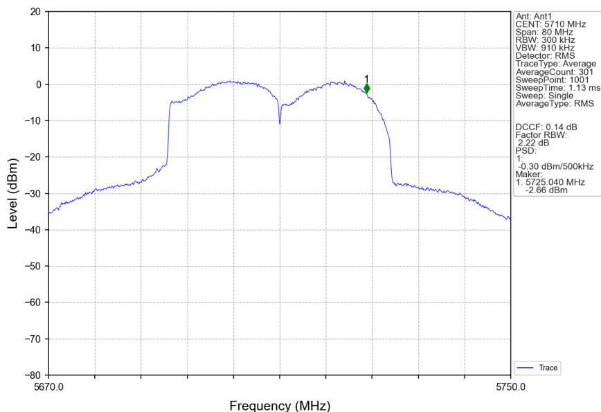
802.11be(EHT40)_HCH_5710MHz_SU_ / _MIMO_NTNV
