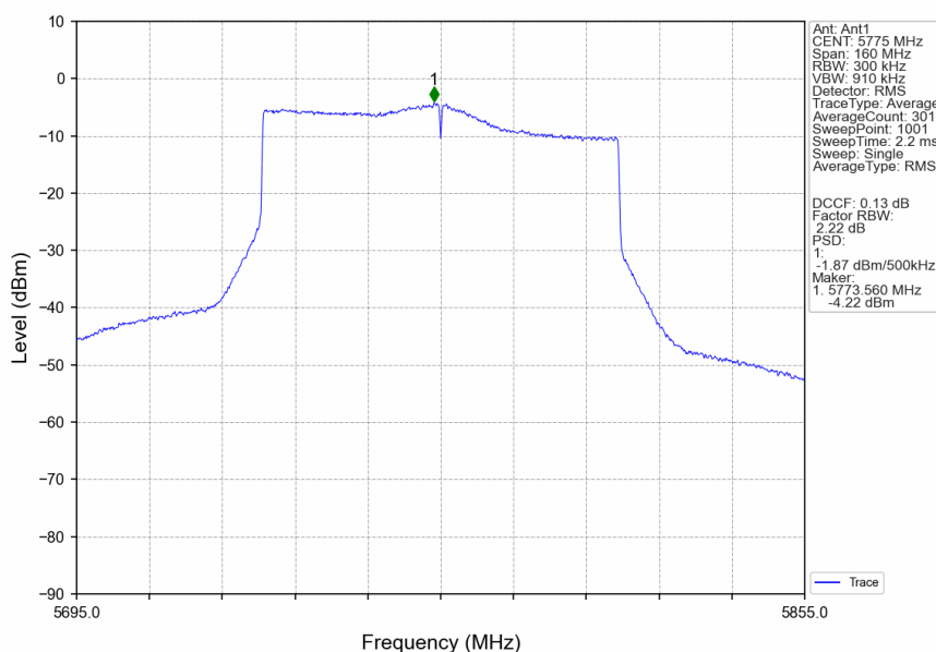
802.11ax(HEW80)_MCH_5775MHz_SU_ / _MIMO_NTNV
