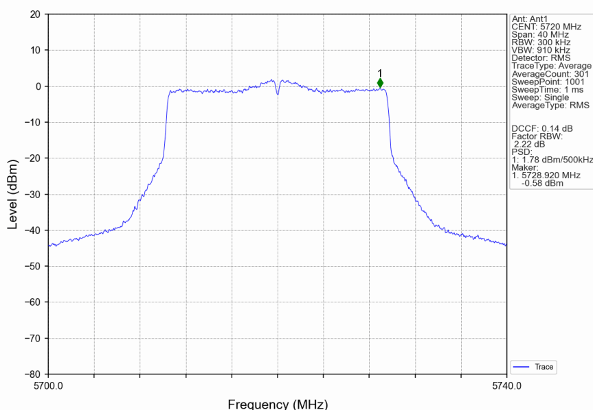
802.11be(EHT20)_HCH_5720MHz_SU_ / _Ant1_NTNV
