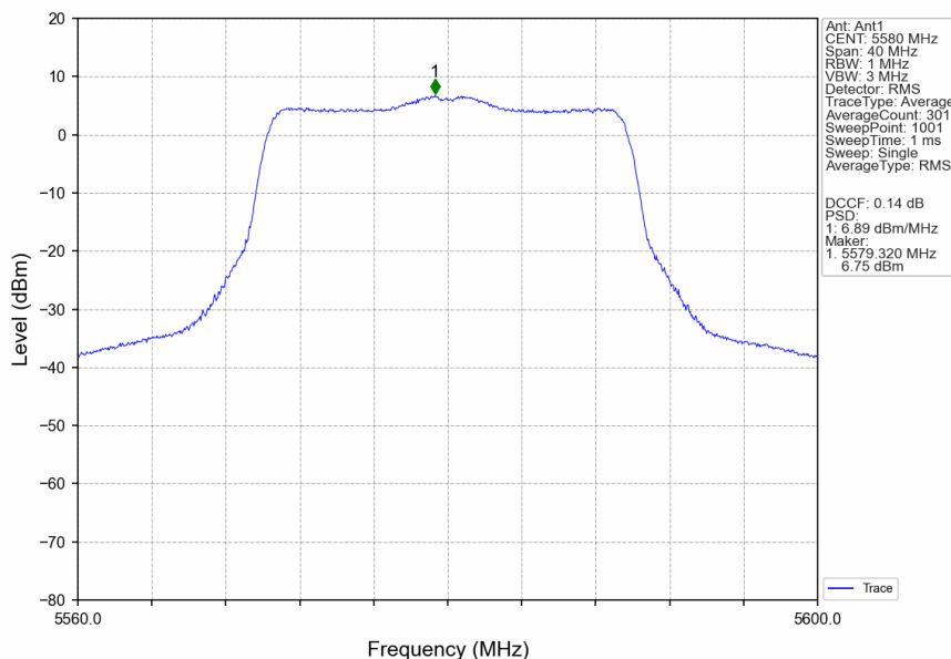
802.11be(EHT20)_MCH_5580MHz_SU_ / _MIMO_NTNV
