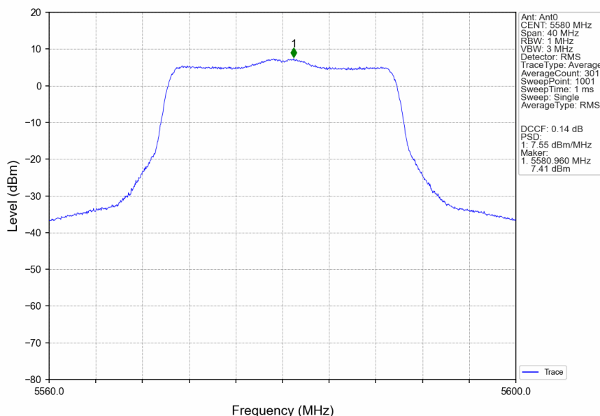
802.11be(EHT20)_MCH_5580MHz_SU_/_Ant0_NTNV
