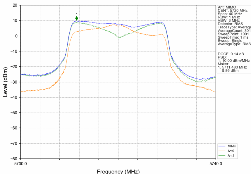
802.11be(EHT20)_HCH_5720MHz_SU_ / _MIMO_NTNV
