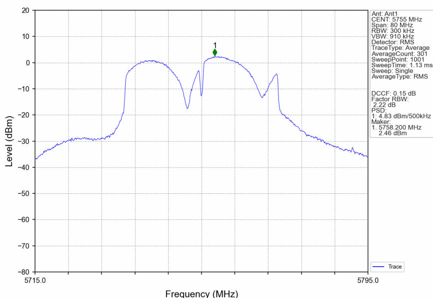
802.11n(HT40)_LCH_5755MHz_Ant1_NTNV
