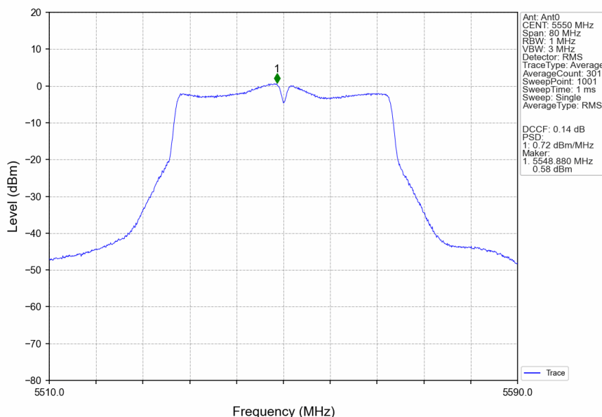
802.11n(HT40)_MCH_5550MHz_Ant0_NTNV
