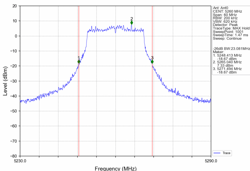
802.11a_LCH_5260MHz_Ant0_NTNV
