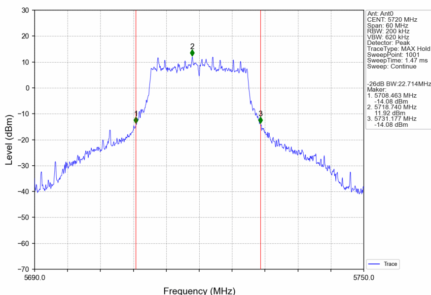
802.11n(HT20)_HCH_5720MHz_Ant0_NTNV
