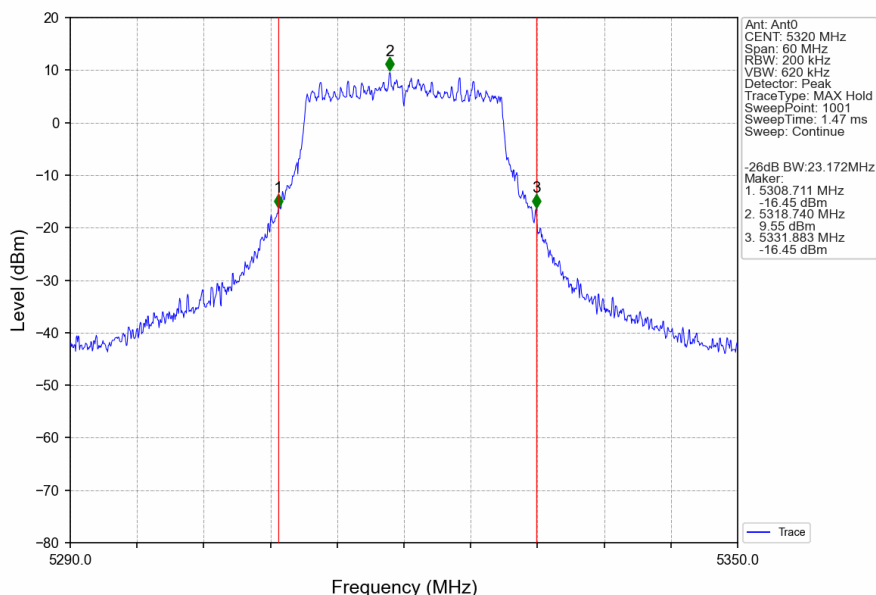
802.11n(HT20)_HCH_5320MHz_Ant0_NTNV
