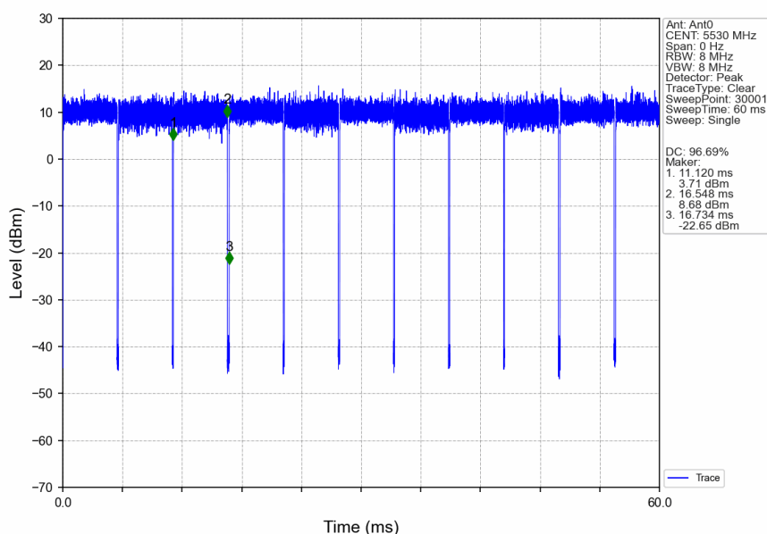
802.11ac(VHT80)_LCH_5530MHz_Ant0_NTNV
