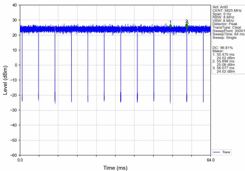
802.11ac(VHT20)_HCH_5825MHz_Ant0_NTNV
