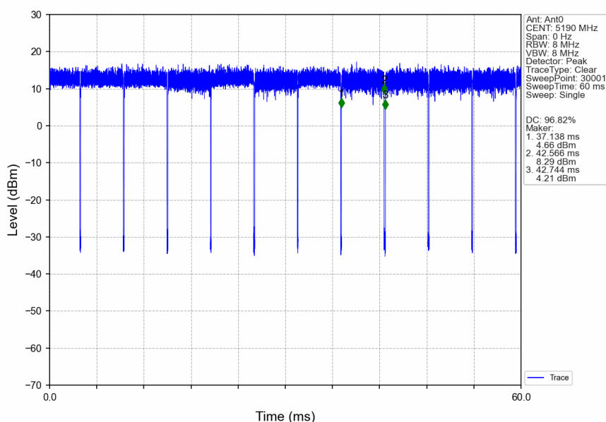
802.11ac(VHT40)_LCH_5190MHz_Ant0_NTNV
