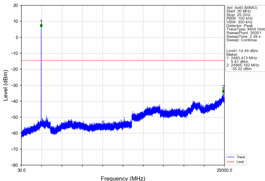
802.11n(HT20)_HCH_2462MHz_Ant0 (MIMO)_NTNV
