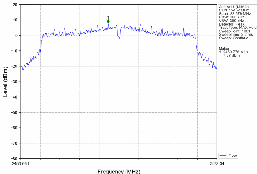
802.11n(HT20)_HCH_2462MHz_Ant1 (MIMO)_NTNV
