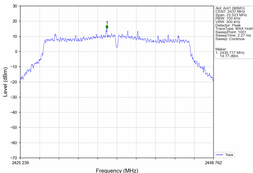
802.11n(HT20)_MCH_2437MHz_Ant1 (MIMO)_NTNV
