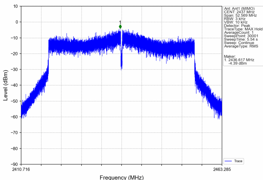
802.11ax(HEW40)_MCH_2437MHz_SU_/_Ant1 (MIMO)_NTNV
