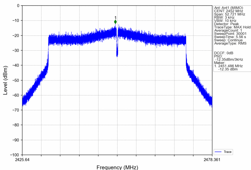
802.11be(EHT40)_HCH_2452MHz_SU_ / _MIMO_NTNV
