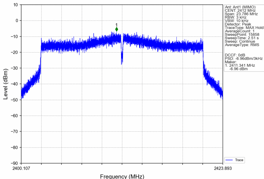
802.11ax(HEW20)_LCH_2412MHz_SU_/_Ant1 (MIMO)_NTNV
