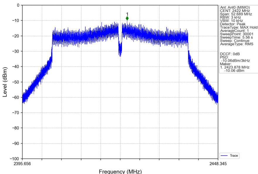
802.11n(HT40)_LCH_2422MHz_Ant0 (MIMO)_NTNV
