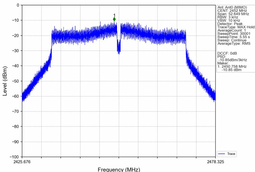
802.11n(HT40)_HCH_2452MHz_Ant0 (MIMO)_NTNV
