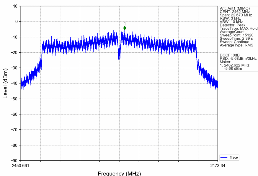
802.11n(HT20)_HCH_2462MHz_Ant1 (MIMO)_NTNV
