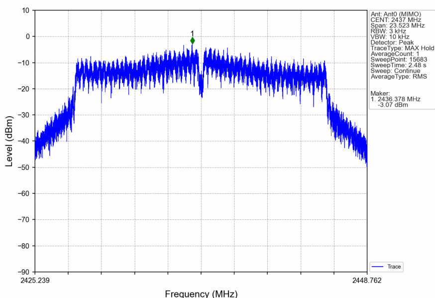
802.11n(HT20)_MCH_2437MHz_Ant0 (MIMO)_NTNV
