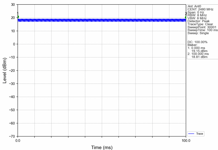
2M_HCH_2480MHz_Ant0_NTNV
