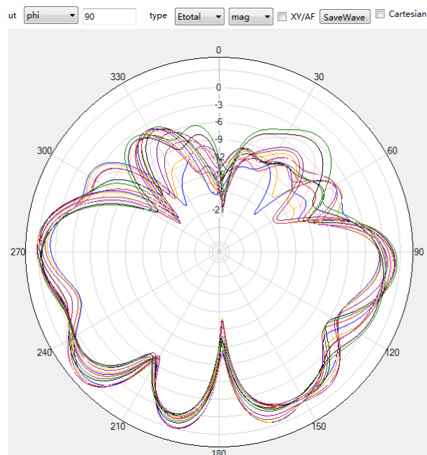
5G phi=90deg
