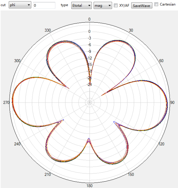
2.4G phi=0deg
