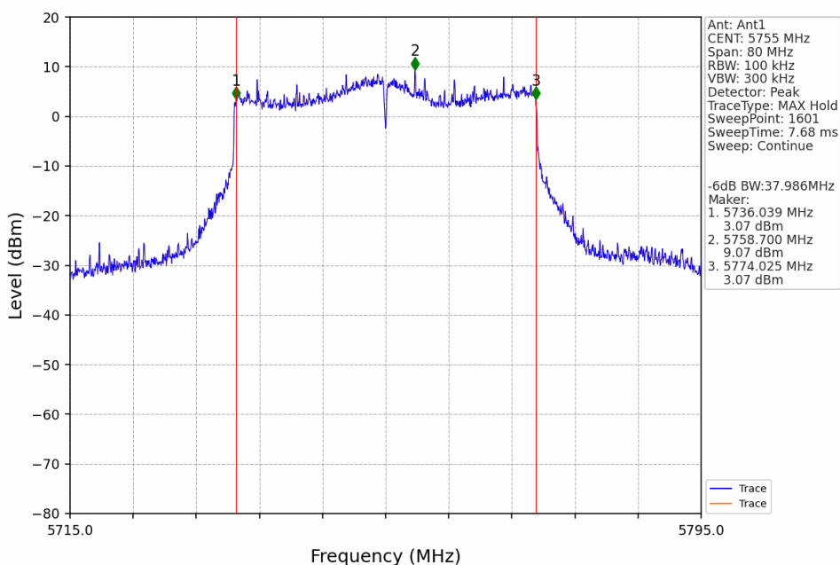
802.11be(EHT40)_LCH_5755MHz_SU_Ant1_NTNV
