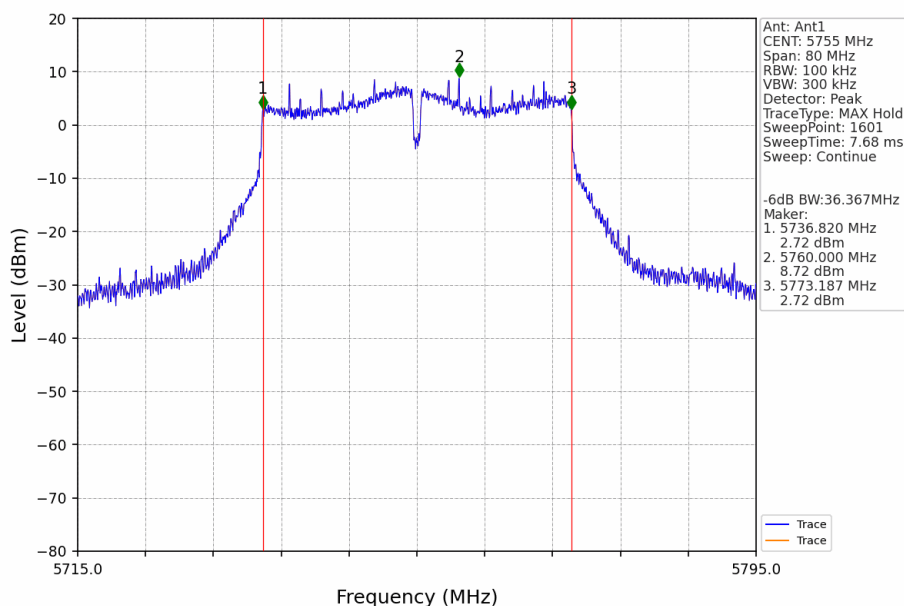
802.11ac(VHT40)_LCH_5755MHz_Ant1_NTNV
