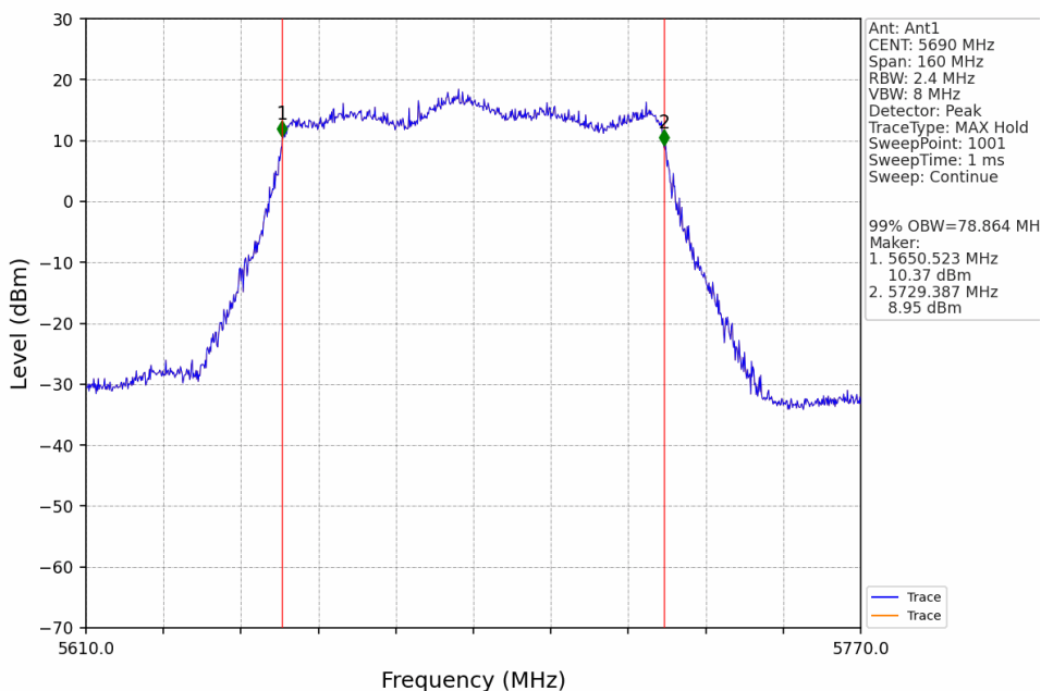
802.11be(EHT80)_HCH_5690MHz_SU_Ant1_NTNV
