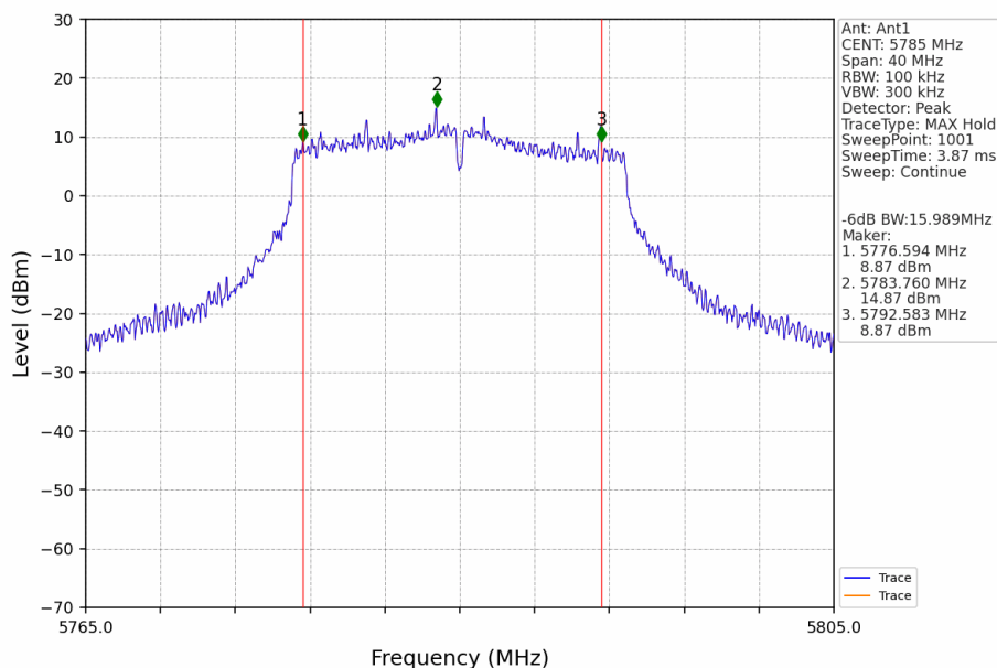
802.11n(HT20)_MCH_5785MHz_Ant1_NTNV
