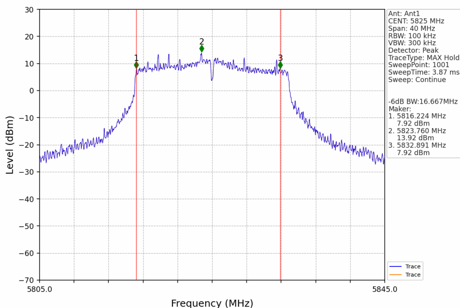
802.11n(HT20)_HCH_5825MHz_Ant1_NTNV
