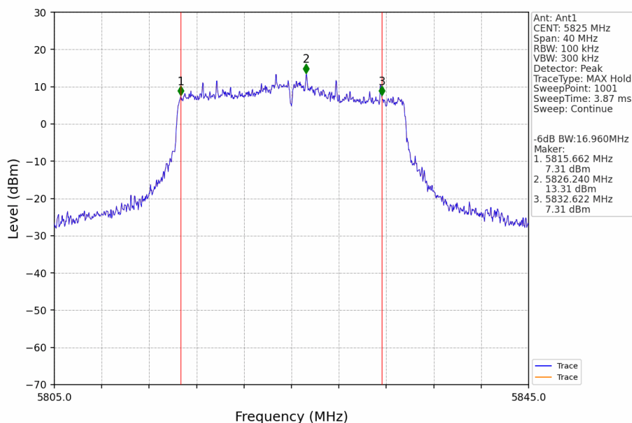
802.11be(EHT20)_HCH_5825MHz_SU_Ant1_NTNV
