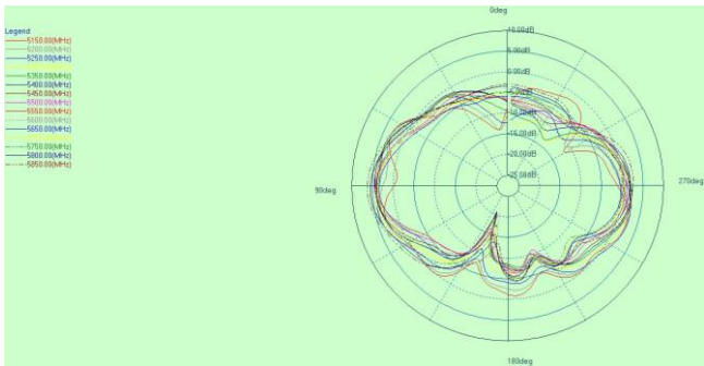
theta=90deg
