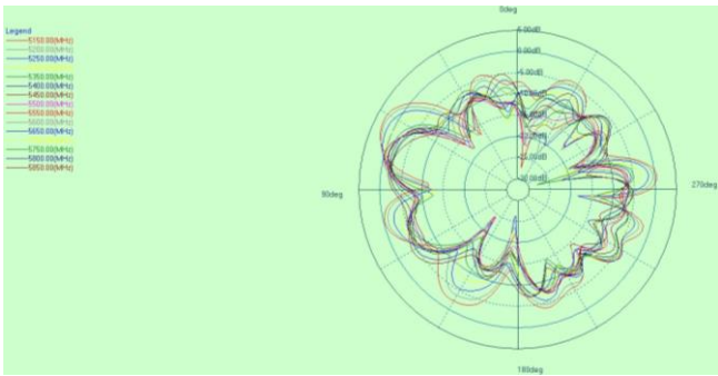
phi=0deg
