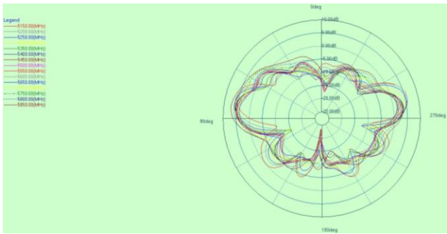
phi=90deg
