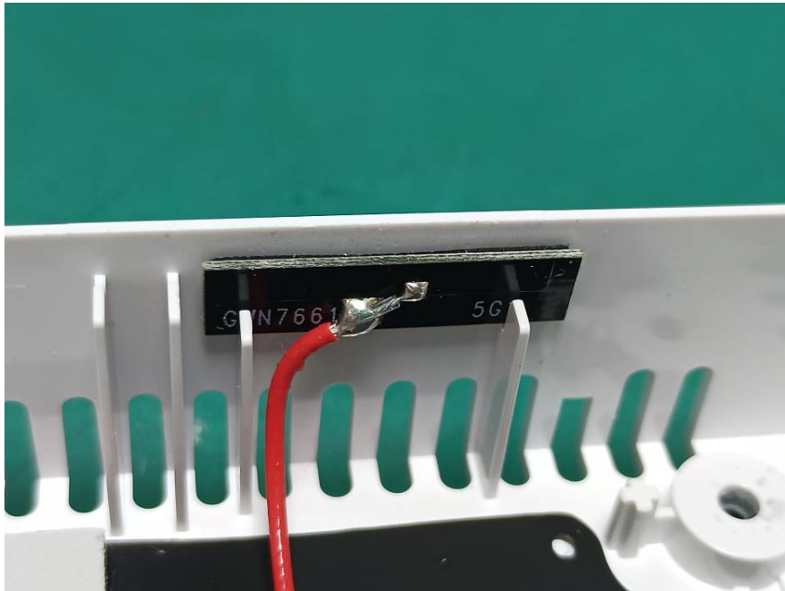
2.4G Wi-Fi ANT1 & 5G Wi-Fi ANT0
