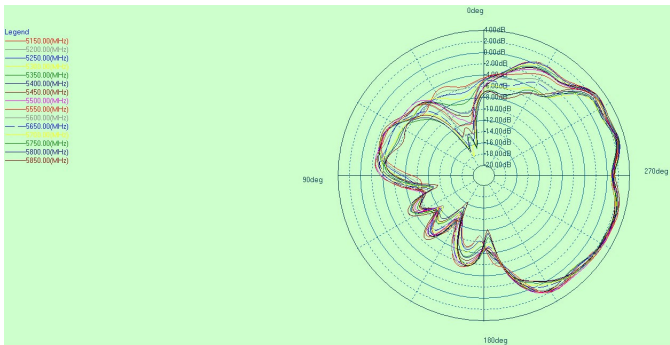
phi=90deg
