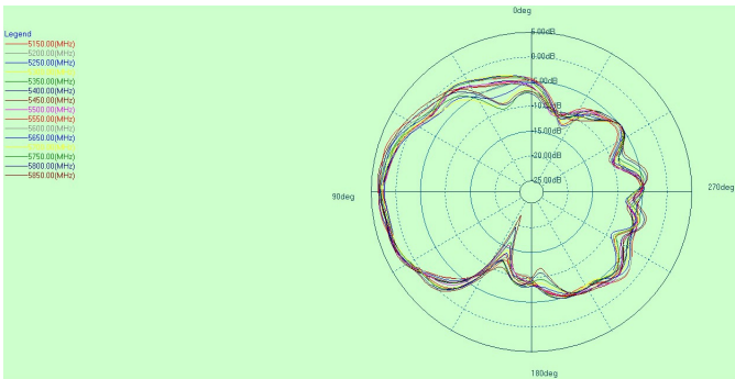
phi=0deg
