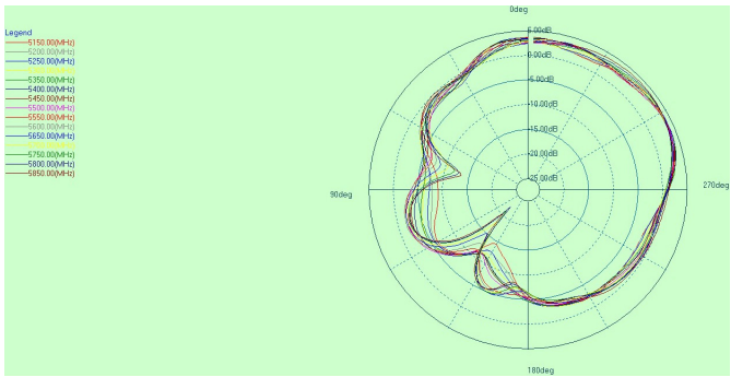
theta=90deg
