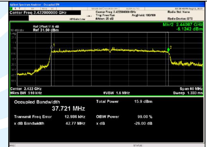
IEEE 802.11ax_Channel 3_40MHz_Antenna 1_RU&amp;Index SU
