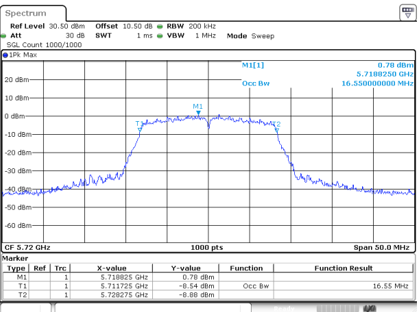
802.11a_5720MHz_Chain 1
