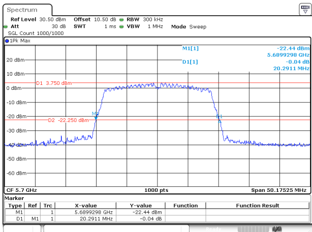
802.11ac20_5700MHz_Chain 0
