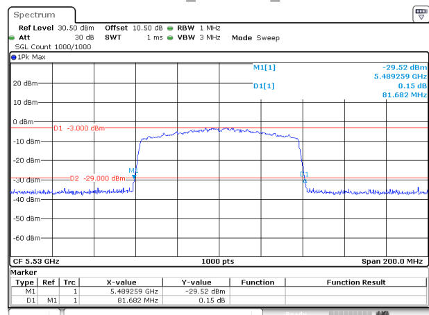
802.11ac80_5530MHz_Chain 1
