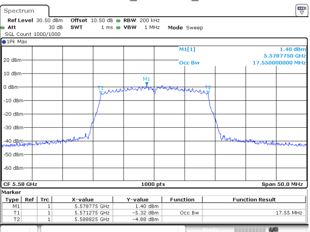
802.11ac20_5580MHz_Chain 0
