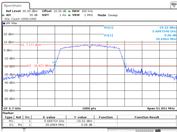
802.11ac20_5700MHz_Chain 1
