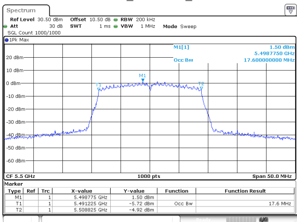
802.11ac20_5500MHz_Chain 0
