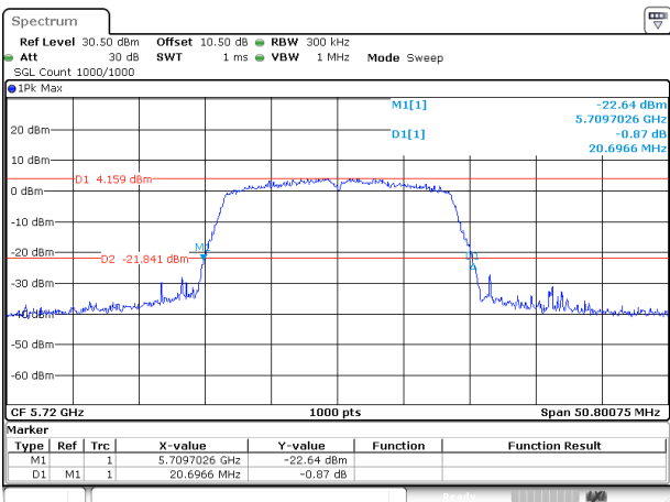
802.11ac20_5720MHz_Chain 1
