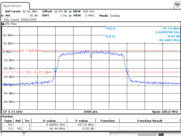
802.11ac40_5710MHz_Chain 0
