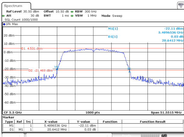
802.11ac20_5500MHz_Chain 1
