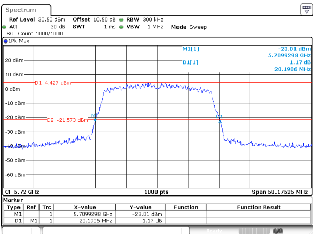
802.11ac20_5720MHz_Chain 0
