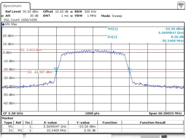
802.11ac20_5580MHz_Chain 0
