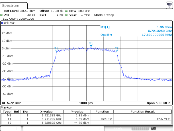
802.11ac20_5720MHz_Chain 0
