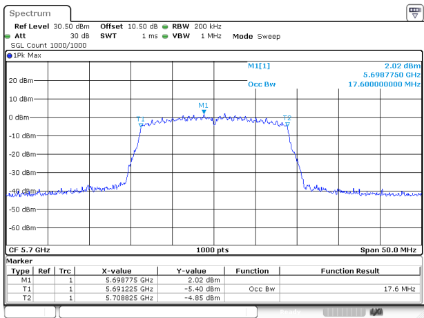
802.11ac20_5700MHz_Chain 0
