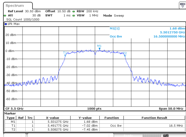
802.11a_5500MHz_Chain 1
