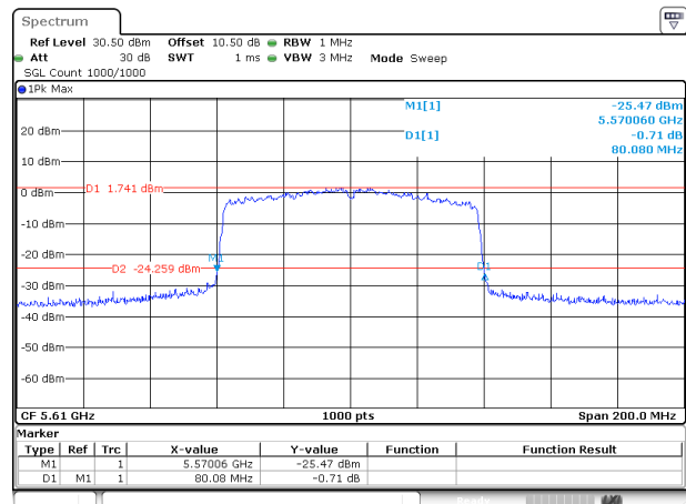
802.11ac80_5610MHz_Chain 0
