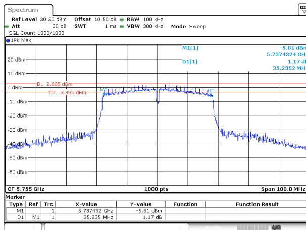
802.11ac40_5755MHz_Chain 1
