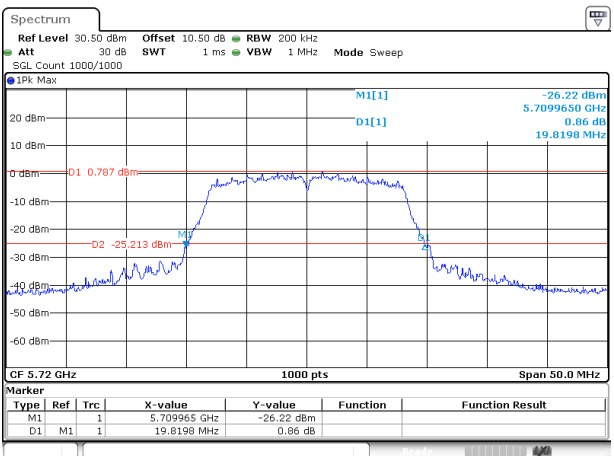
802.11a_5720MHz_Chain 1
