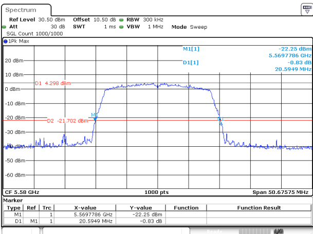
802.11ac20_5580MHz_Chain 1
