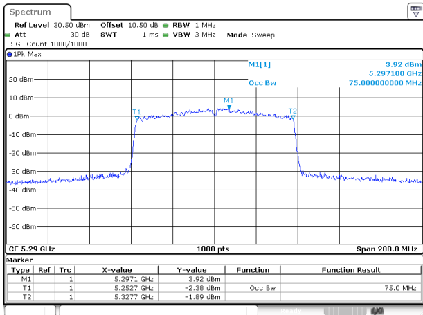
802.11ac80_5290MHz_Chain 0
