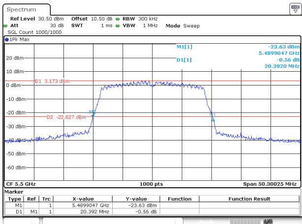
802.11ac20_5500MHz_Chain 0
