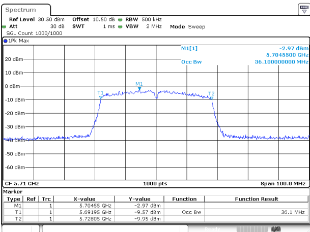
802.11ac40_5710MHz_Chain 1
