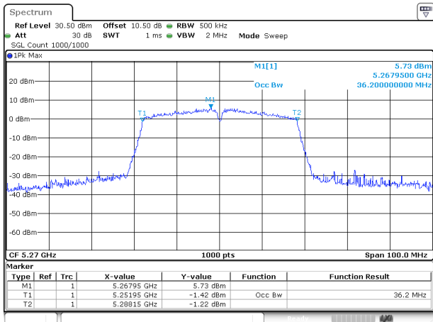
802.11ac40_5270MHz_Chain 1
