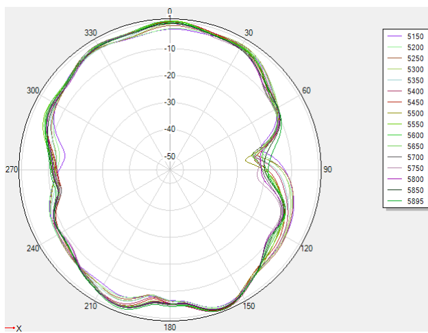
5G phi=0deg
