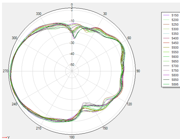
5G theta=90deg
