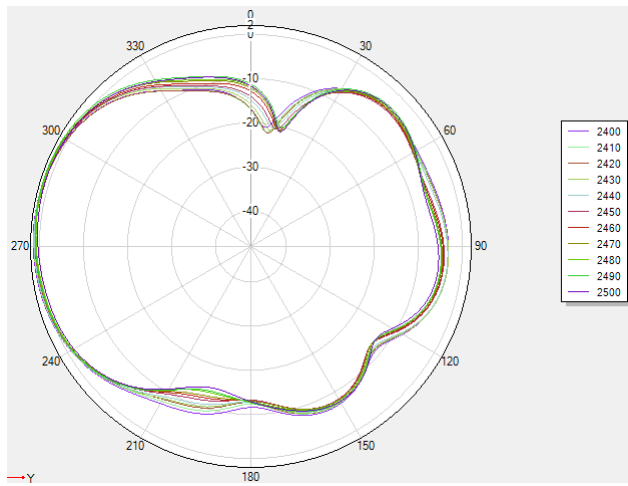
2.4G theta=90deg
