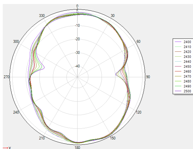
2.4G phi=0deg
