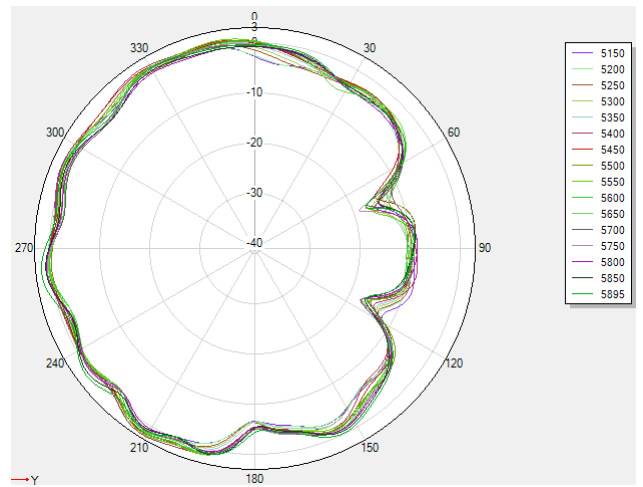
5G phi=90deg
