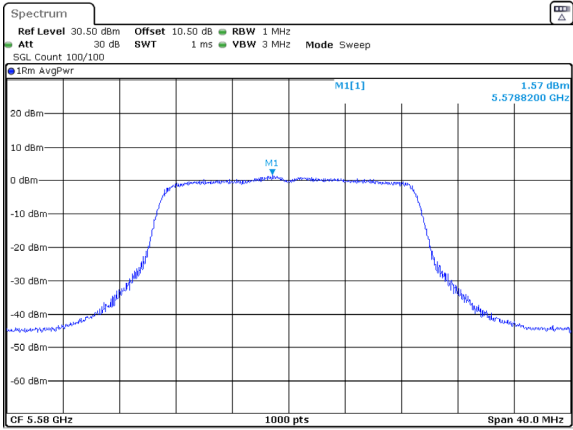
802.11ac20_5580MHz_Chain 1
