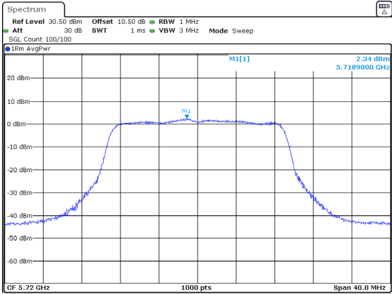
802.11ac20_5720MHz_Chain 1
