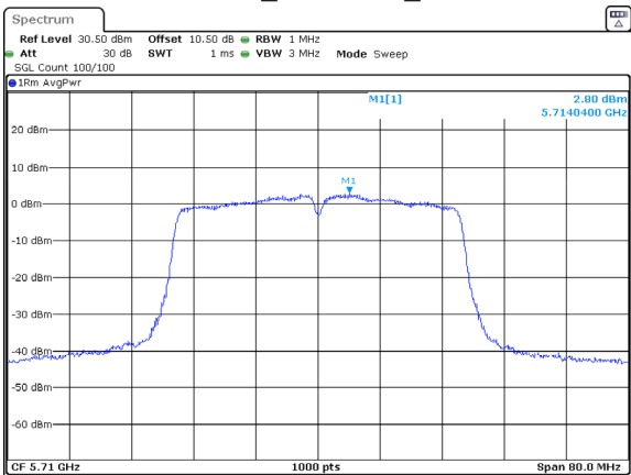
802.11ac40_5710MHz_Chain 1
