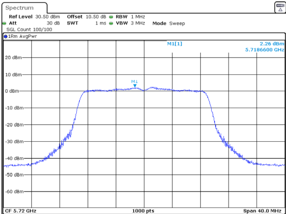
802.11ac20_5720MHz_Chain 0
