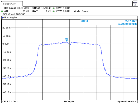
802.11ac40_5710MHz_Chain 0
