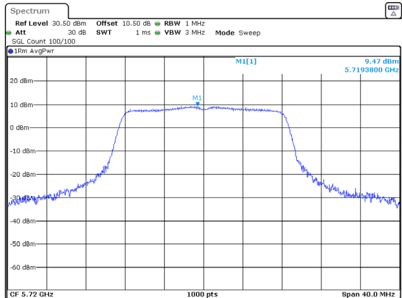
802.11a_5720MHz_Chain 2
