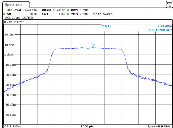
802.11a_5500MHz_Chain 2
