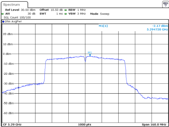
802.11ac80_5290MHz_Chain 2
