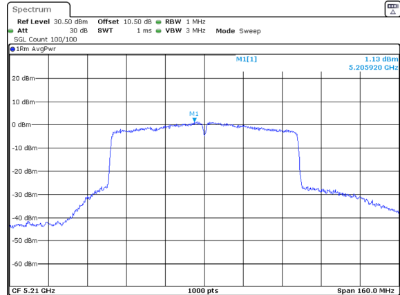
802.11ac80_5210MHz_Chain 1
