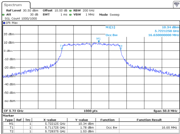
802.11a_5720MHz_Chain 2
