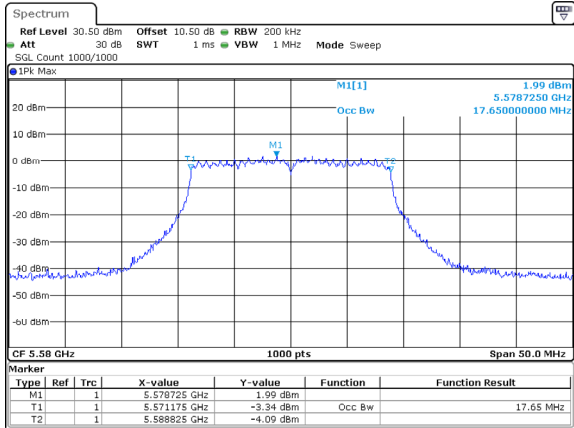
802.11ac20_5580MHz_Chain 1
