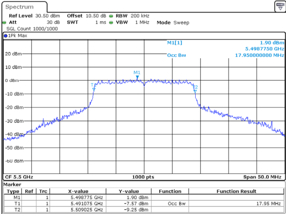
802.11ac20_5500MHz_Chain 1
