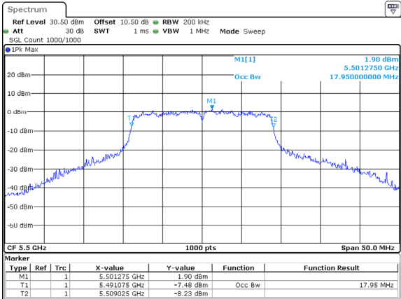
802.11ac20_5500MHz_Chain 0
