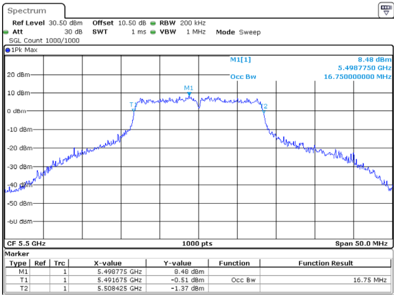
802.11a_5500MHz_Chain 2
