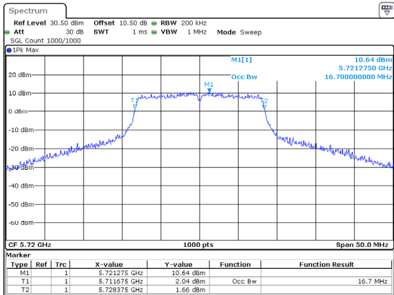
802.11a_5720MHz_Chain 1
