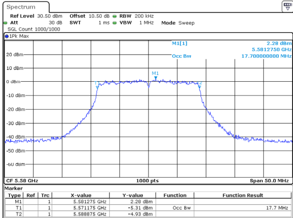
802.11ac20_5580MHz_Chain 0
