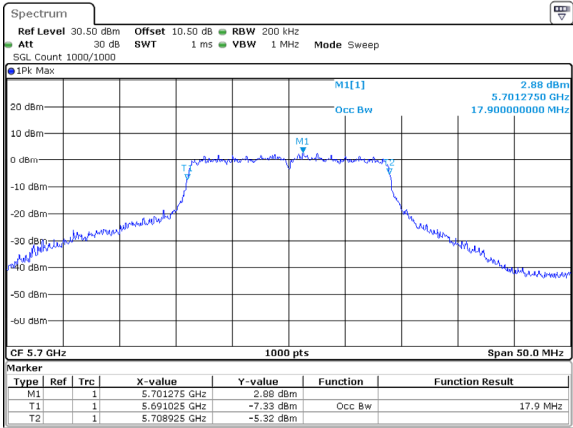
802.11ac20_5700MHz_Chain 0
