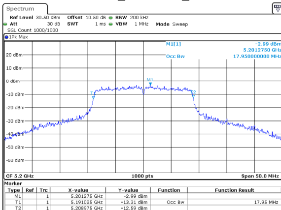
802.11ac20_5200MHz_Chain 0
