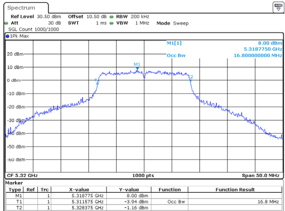
802.11a_5320MHz_Chain 2
