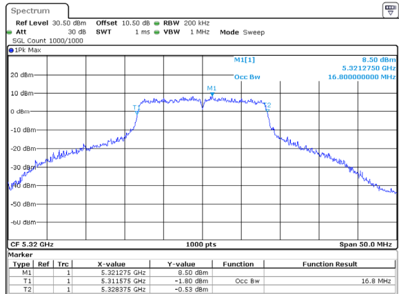
802.11a_5320MHz_Chain 1
