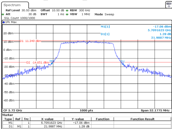
802.11a_5720MHz_Chain 0 21.989MHz
