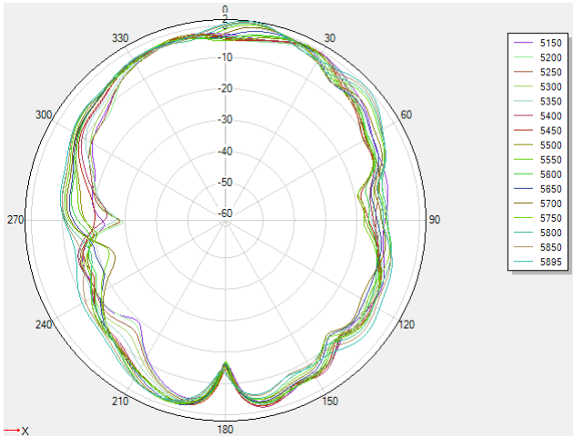
phi=0deg
