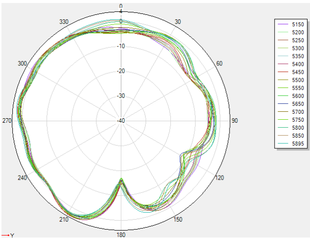
phi=90deg
