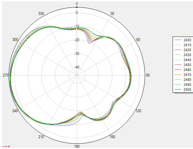
2.4G theta=90deg
