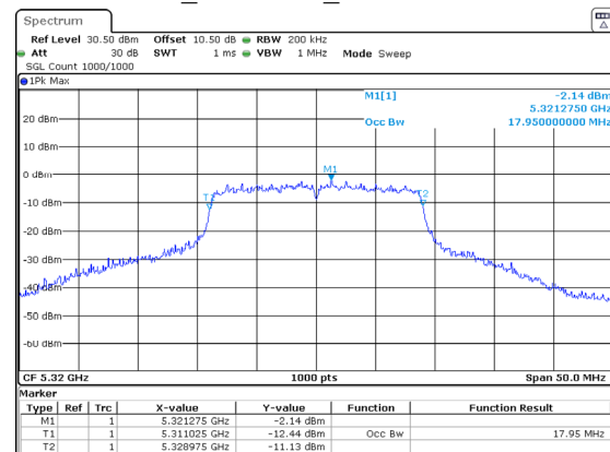
802.11ac20_5320MHz_Chain 0 17.950MHz
