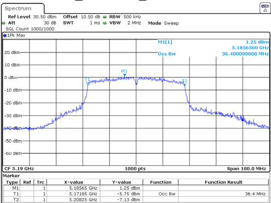
802.11ac40_5190MHz_Chain 2 36.400MHz
