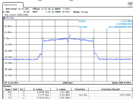
802.11ac160_5250MHz_Chain 2 154.400MHz
