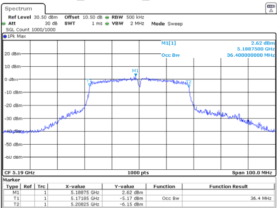
802.11ac40_5190MHz_Chain 1 36.400MHz
