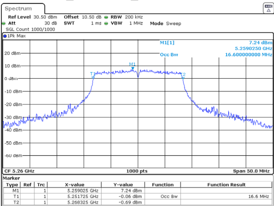
802.11a_5260MHz_Chain 2 16.600MHz
