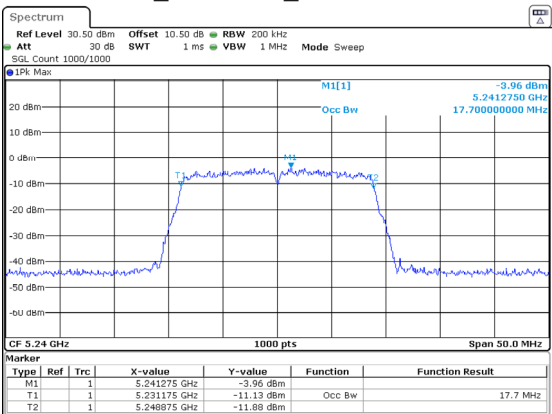
802.11ac20_5240MHz_Chain 0 17.700MHz
