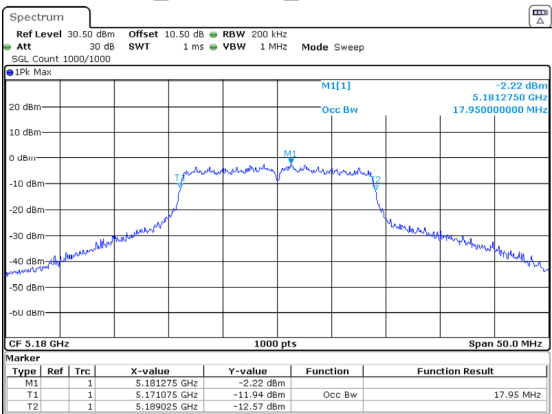
802.11ac20_5180MHz_Chain 0 17.950MHz
