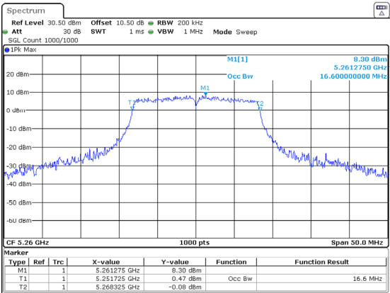
802.11a_5260MHz_Chain 1 16.600MHz
