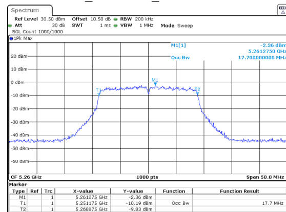
802.11ac20_5260MHz_Chain 0 17.700MHz
