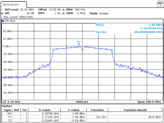
802.11ac40_5190MHz_Chain 0 36.600MHz
