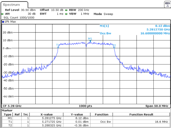
802.11a_5280MHz_Chain 1 16.600MHz
