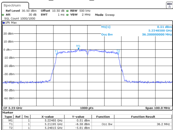
802.11ac40_5230MHz_Chain 2 36.200MHz
