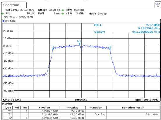
802.11ac40_5230MHz_Chain 1 36.100MHz
