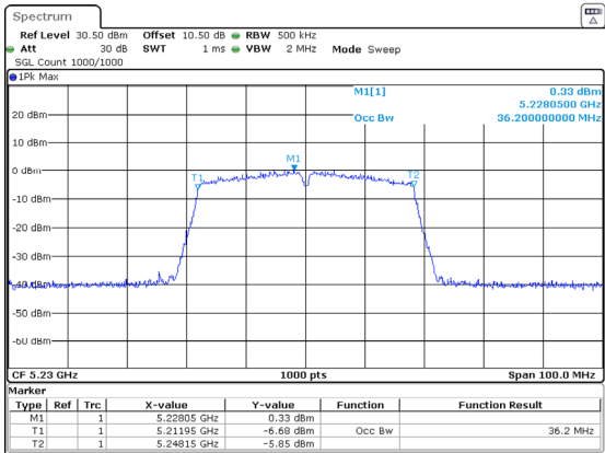
802.11ac40_5230MHz_Chain 0 36.200MHz
