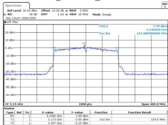
802.11ac160_5250MHz_Chain 0 154MHz
