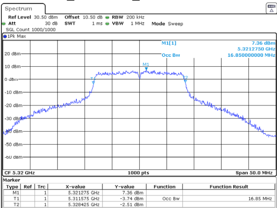
802.11a_5320MHz_Chain 2 16.850MHz
