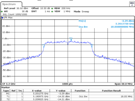
802.11ac20_5200MHz_Chain 0 18.050MHz
