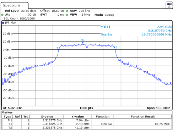
802.11a_5320MHz_Chain 1 16.750MHz
