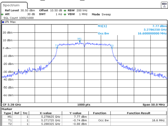
802.11a_5280MHz_Chain 2 16.600MHz
