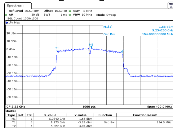
802.11ac160_5250MHz_Chain 1 154MHz
