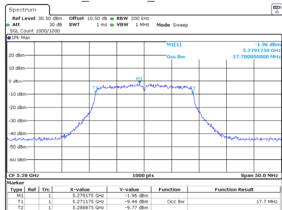
802.11ac20_5280MHz_Chain 0 17.700MHz
