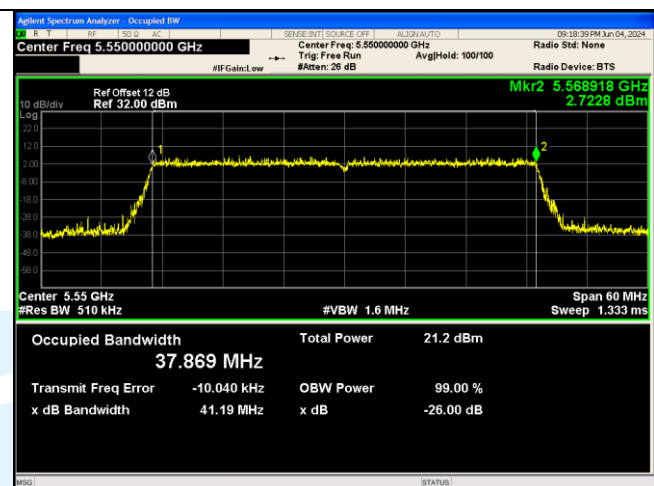
IEEE 802.11ax_Channel 110_40MHz_Antenna 0_RU&Index SU
