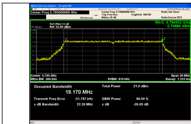
IEEE 802.11ax_Channel 157_20MHz_Antenna 0_RU&amp;Index SU
