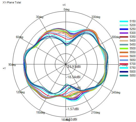
5G theta=90deg
