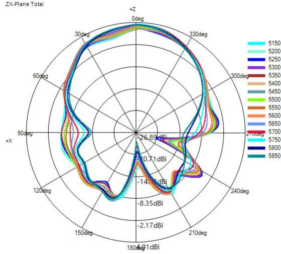
5G phi=0deg
