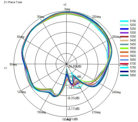
5G phi=90deg
