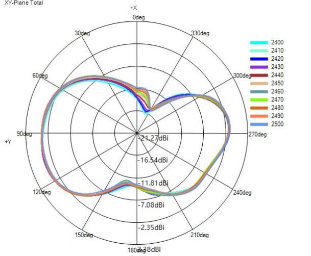
2.4G theta=90deg
