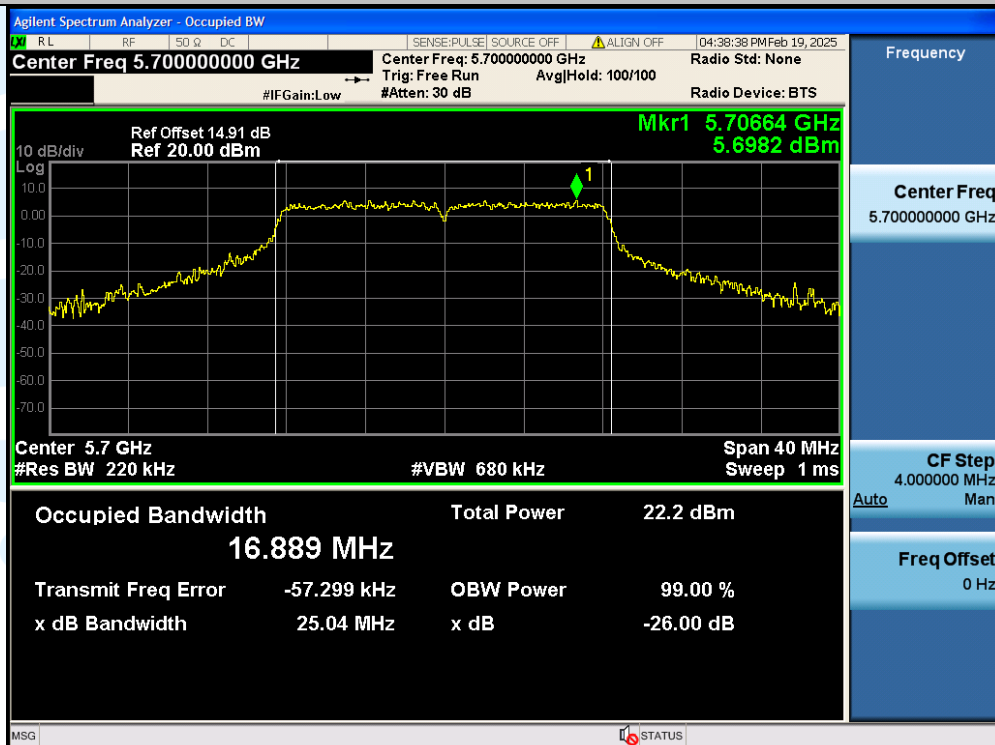
11A-Ant1-5700
