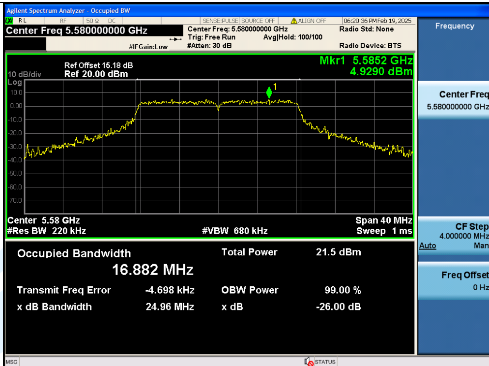
11A-Ant1-5580
