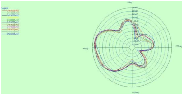
2.4G theta=90deg
