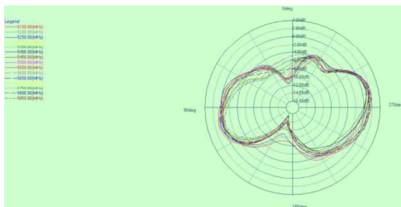
5G theta=90deg
