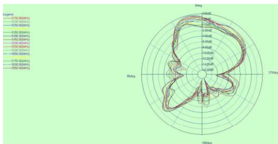
5G phi=0deg
