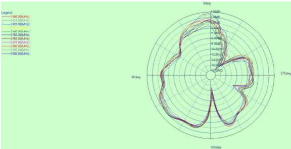
2.4G phi=0deg
