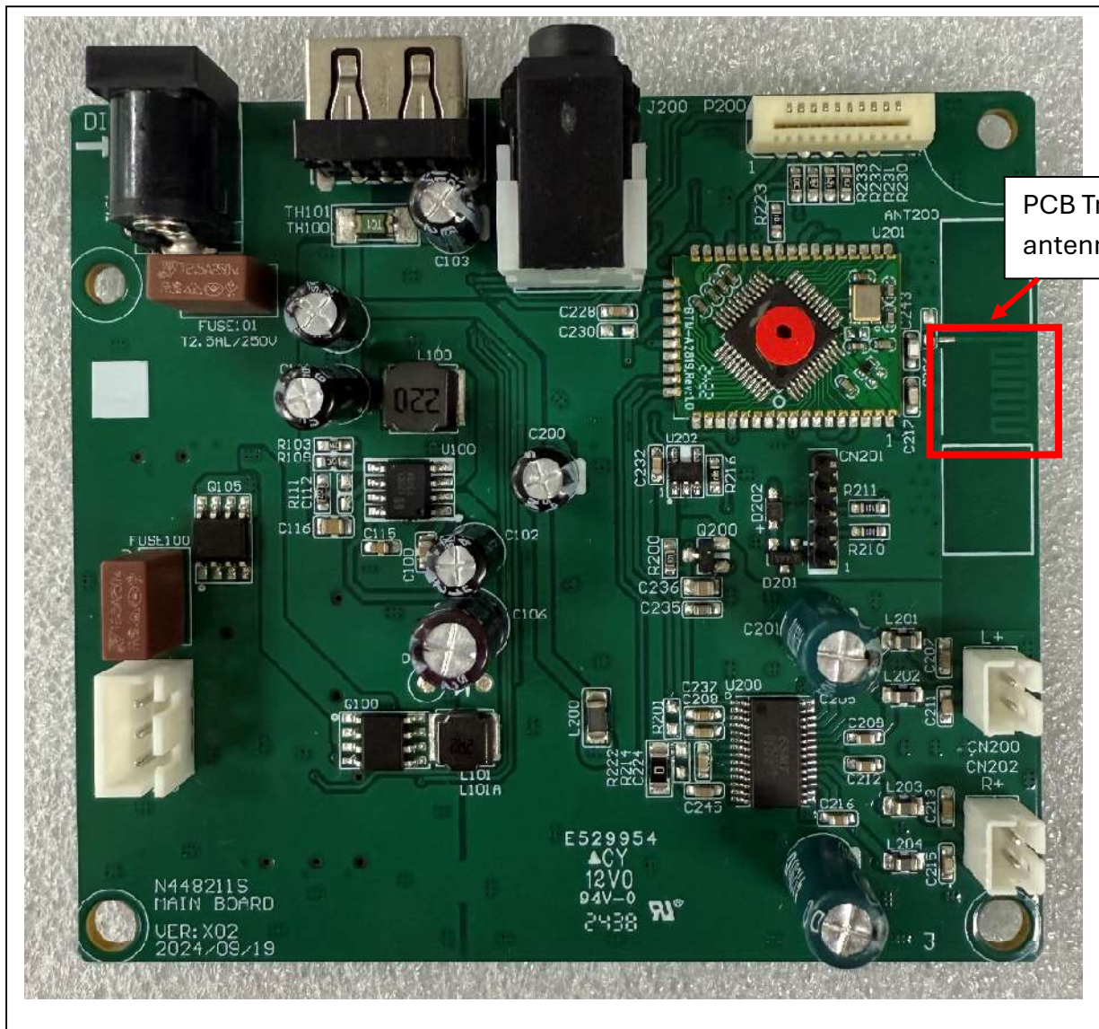
Main PCA – Top
