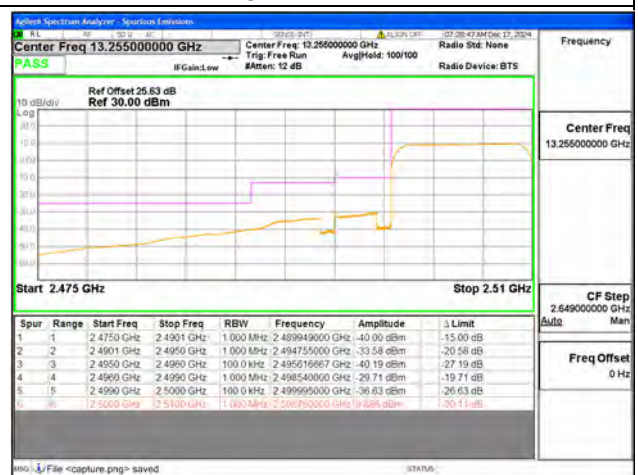
B7 / 10MHz / Low CH / QPSK / FULL RB
