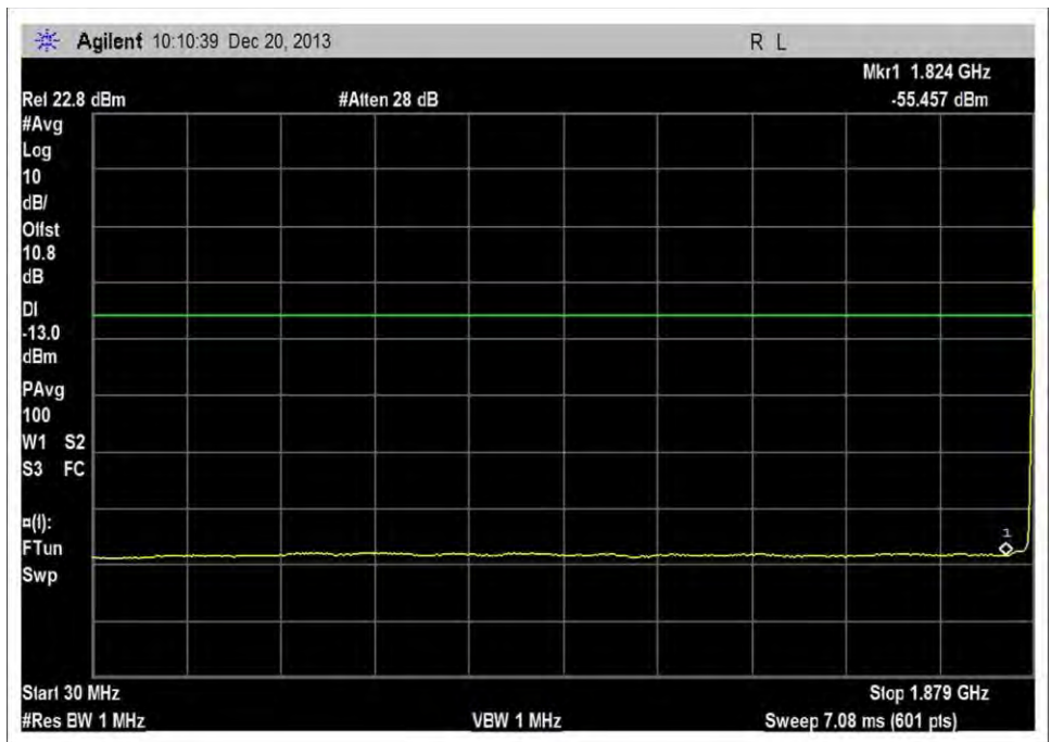
UL_1850-1915MHz_M_5WCDMATM1_2
