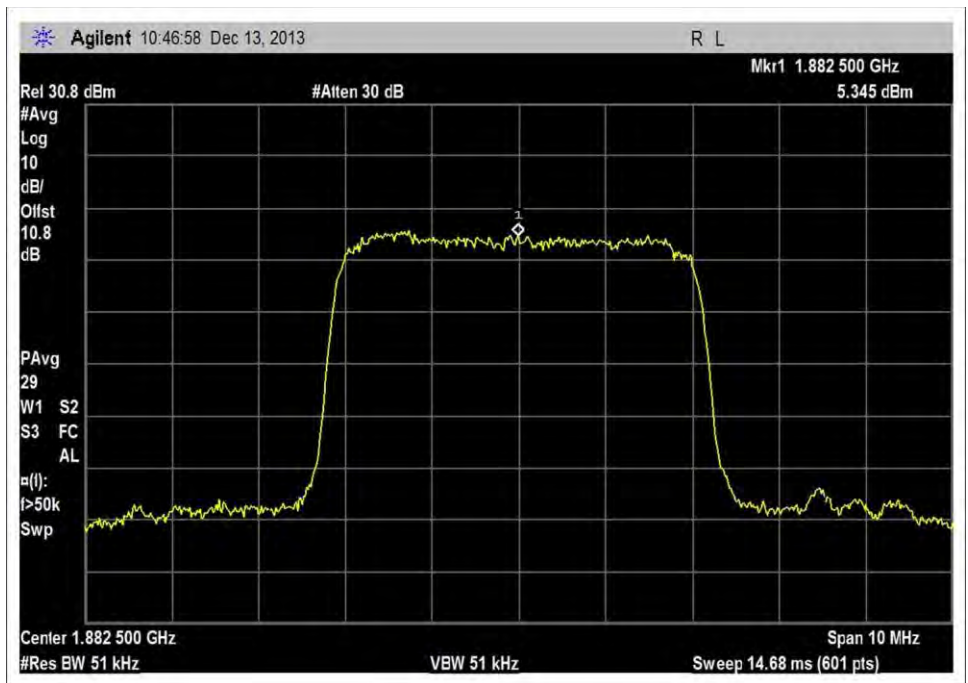
UL_1850-1915MHz_Output
