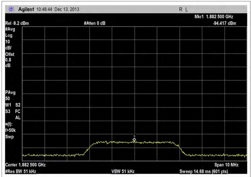
UL_1850-1915MHz_Input
