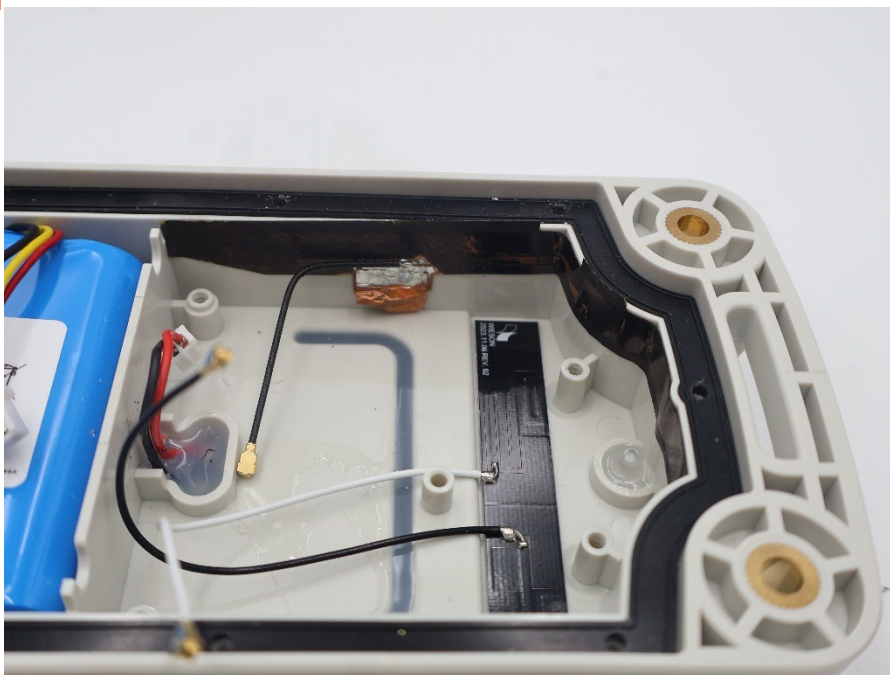
GPS RFIC
