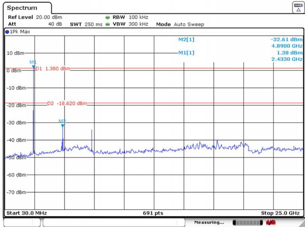
GFSK 2441 MHz
