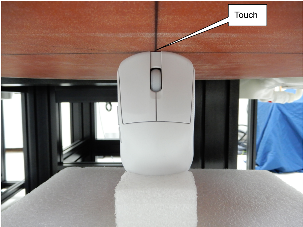
EUT Top
