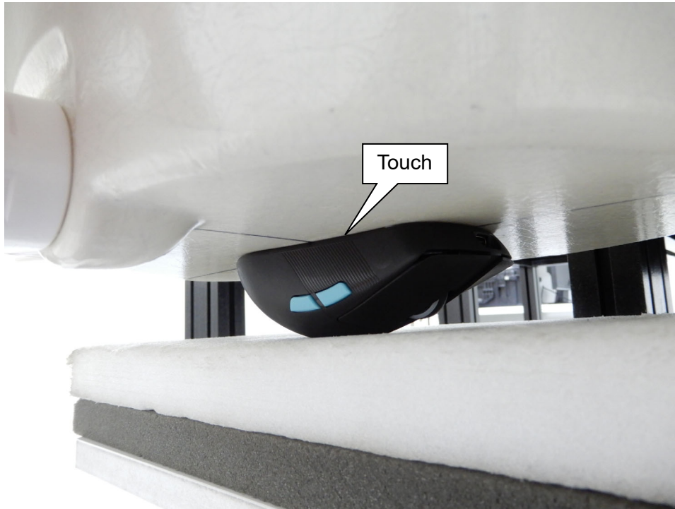
EUT Back
