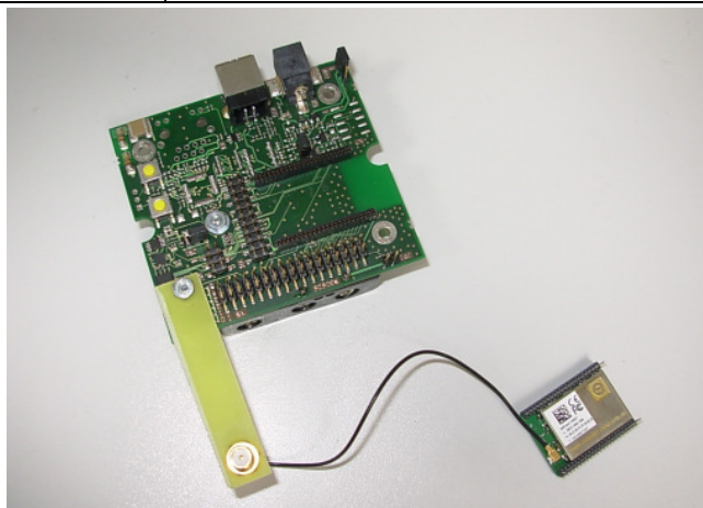
Figure 5: Test sample with disconnected radio module [Prüfmuster mit abgezogenem Funkmodul]
