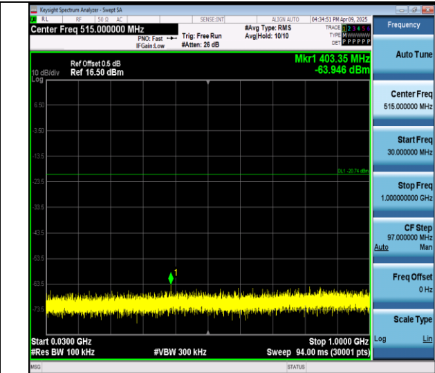
BLE 1M-Ant0-2402-30~1000-PASS
