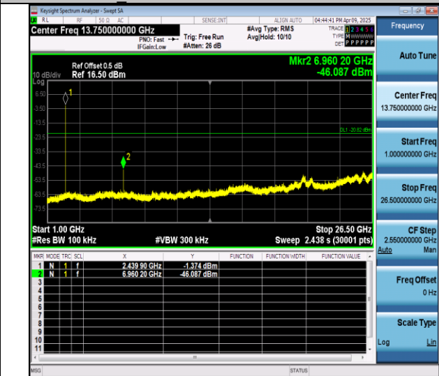
BLE 1M-Ant0-2440-1000~26500-PASS
