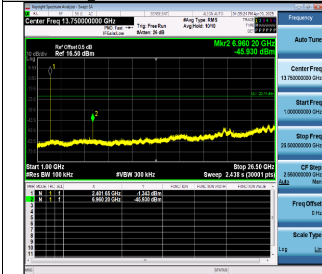
BLE 1M-Ant0-2402-1000~26500-PASS
