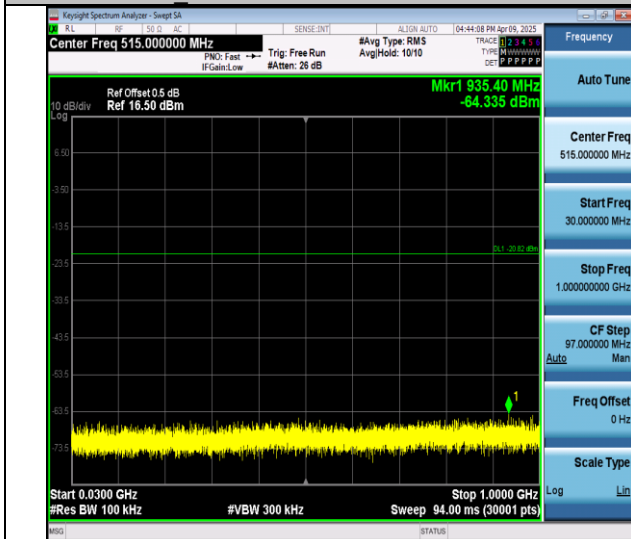
BLE 1M-Ant0-2440-30~1000-PASS
