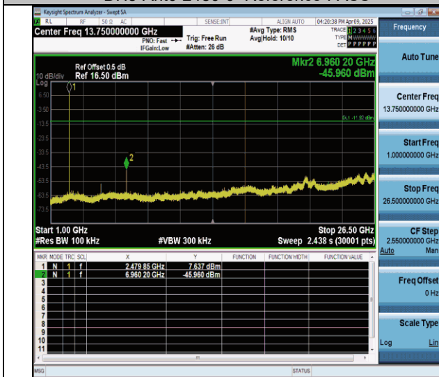
DH5-Ant0-2480-1000~26500-PASS
