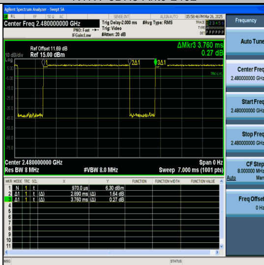
NTNV-3DH5-Ant0-2480
