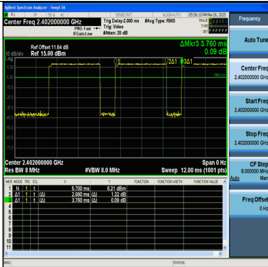
NTNV-3DH5-Ant0-2402
