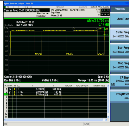
NTNV-3DH5-Ant0-2441
