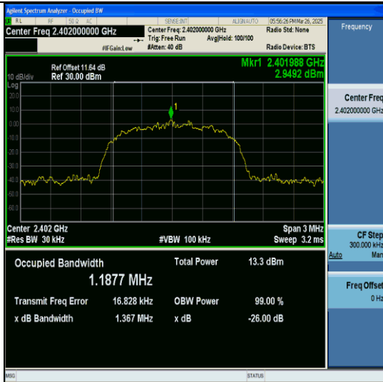
3DH5-Ant0-2402
