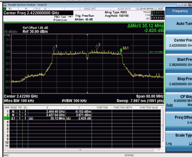
11n40SISO-Ant0-2422-PASS
