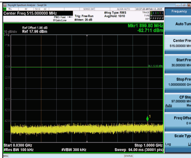
11b-Ant0-2462-30~1000-PASS
