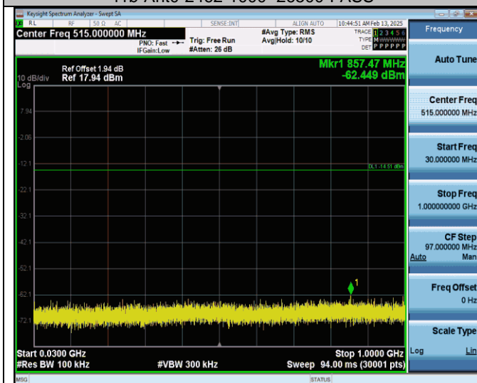
11g-Ant0-2412-30~1000-PASS
