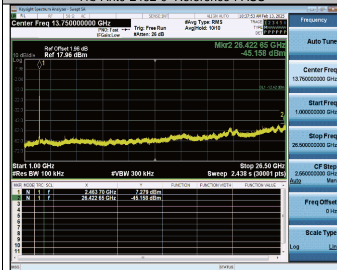
11b-Ant0-2462-1000~26500-PASS
