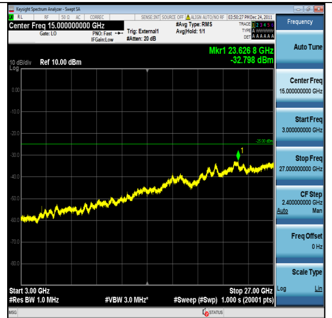
Band41-20MHz-QPSK-39750-1RB#0-3000~27000-PASS
