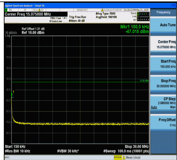
GSM1900-512-0-0.15~30MHz-PASS
