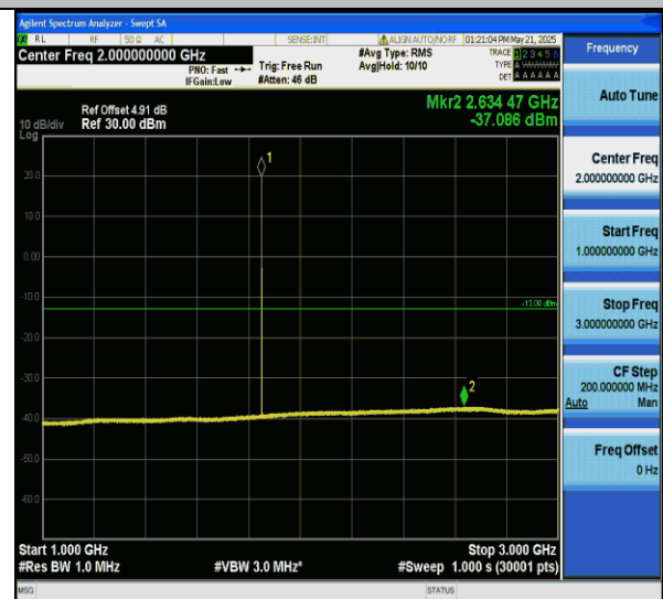
GSM1900-512-0-1000~3000MHz-PASS
