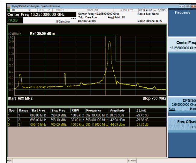
Band71-10MHz-QPSK-133422-1RB#49-PASS
