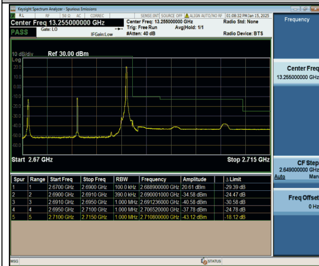
Band41-20MHz-QPSK-41490-1RB#99-PASS
