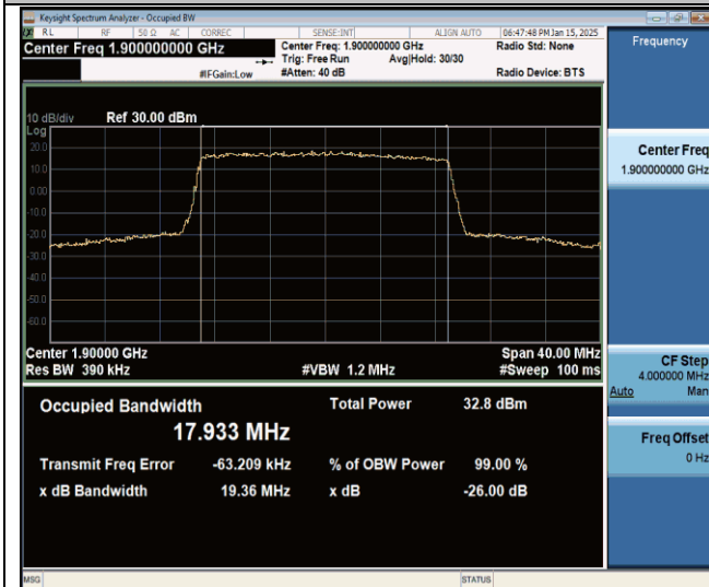
Band2-20MHz-QPSK-19100-100RB#0-PASS
