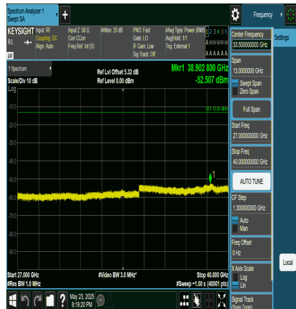
NTNV_N77-3700- 3980_PC2_30_20_L_TID2_NS_01_27000_40000_#1
