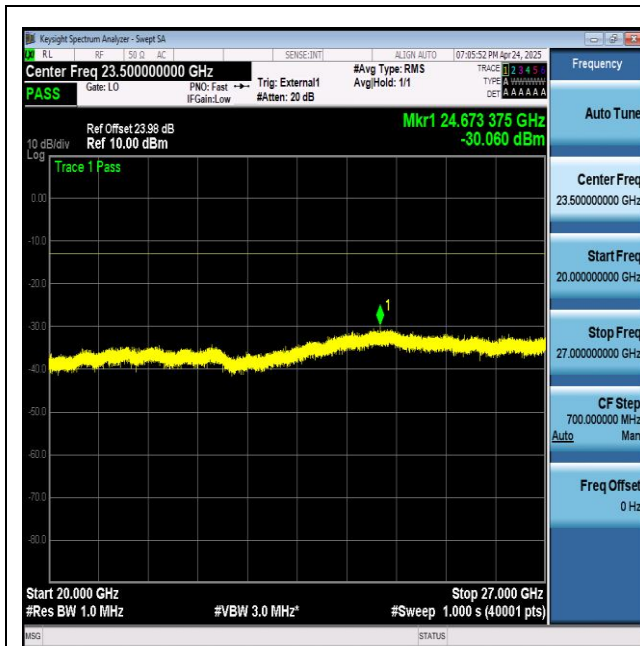
NTNV_N77-3700- 3980_PC2_30_20_L_TID2_NS_01_20000_27000_#1
