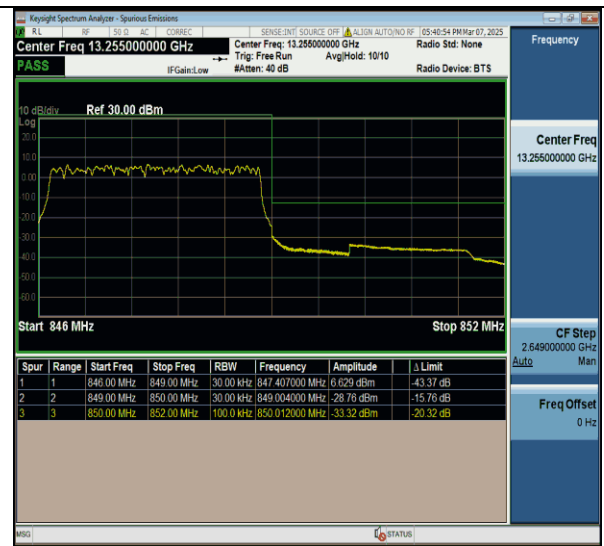
Band26(824-849)-3MHz-QSPK-27025-15RB#0-PASS
