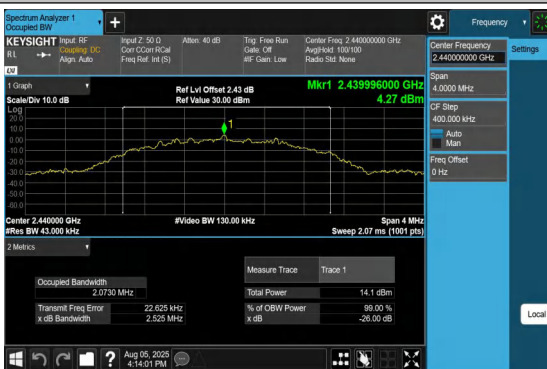
BLE_2M-Ant1-2440
