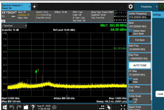
BLE_2M-Ant1-2480-30~1000-PASS
