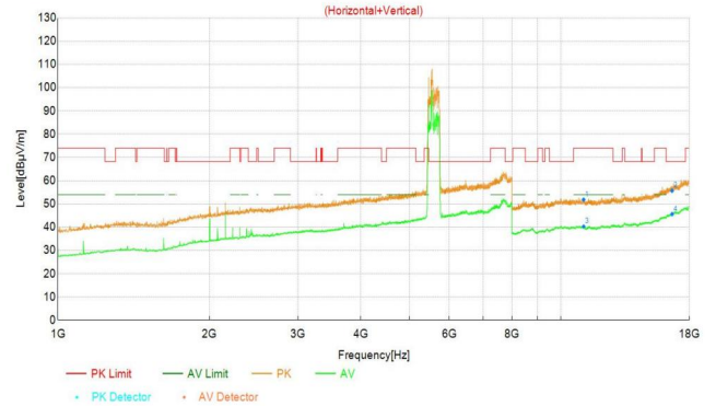
11N_40M_5710
